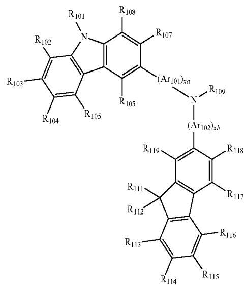
HMTPD
