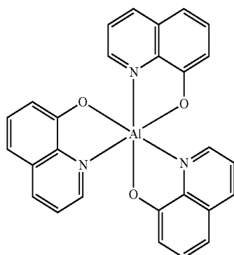
Alq 3
